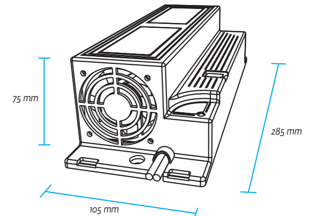
peso | weight | Gewicht | peso: 1.39 kg
